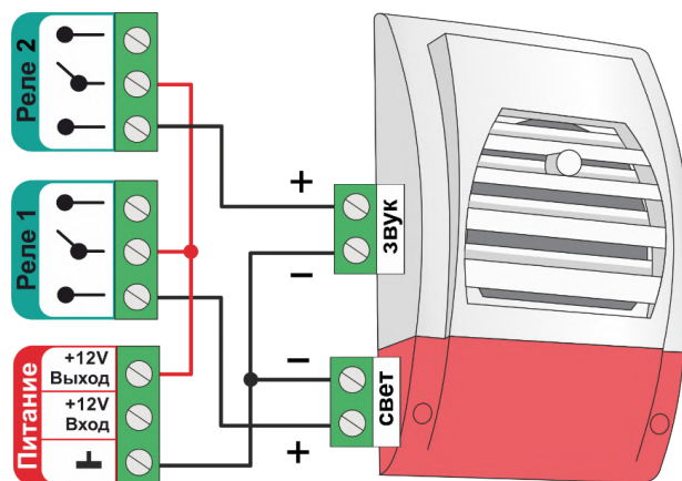
Схема подключения свето-звукового оповещателя к релейному выходу
